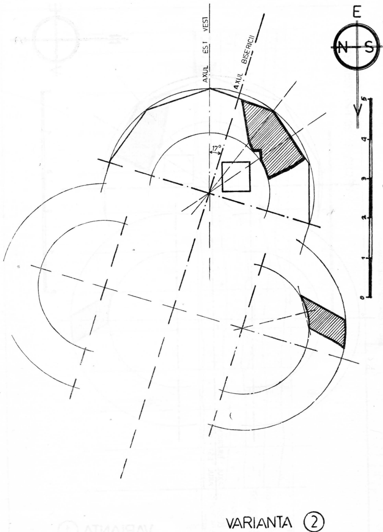
Fig. 3. Ghica-Tei, Planul bisericii, Varianta 2.
